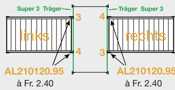
Kit T Verbindungsklammern, für links und rechts verwendbar
