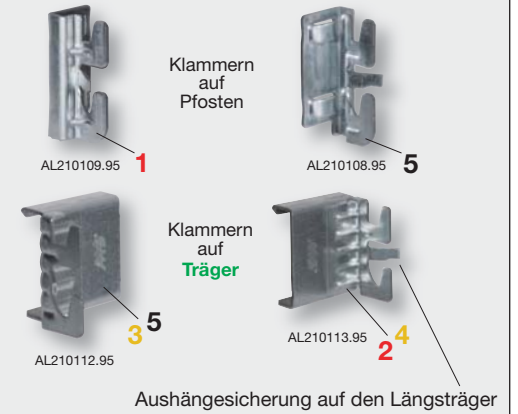
Aushängesicherung auf den Längsträger
