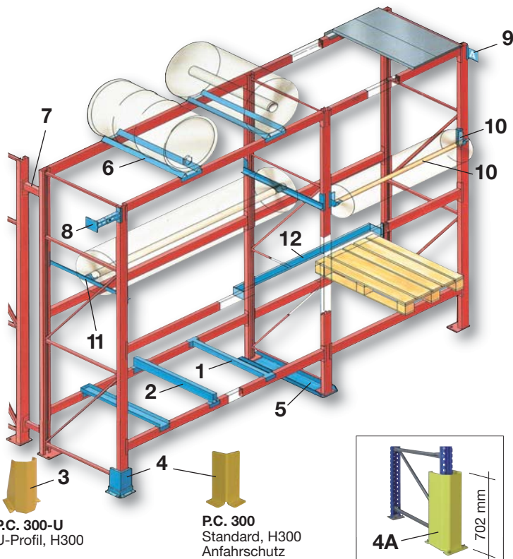
PC. 300-U-PL für Weitspannregale / Plattformen, H702
