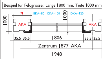
Paneelen, siehe Blatt 13.5 Pos.15 / ZR 06
