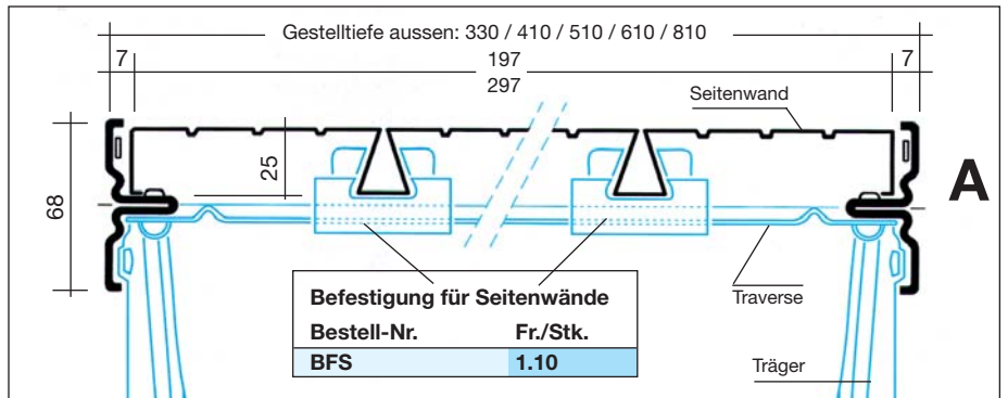
Information über die Montage von Seitenwänden. Dargestellt eine Seitenwand mit Profilierung 25 mm. Bestell-Nr. und Preise der Seitenwände, siehe Blatt 10.11
