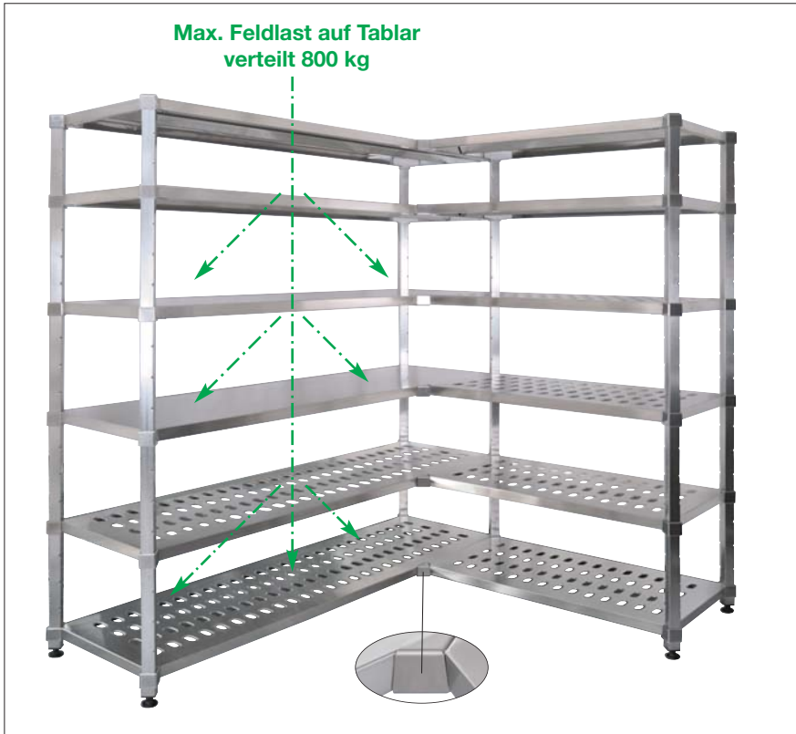
Eckverbindungen siehe auf Blatt 12.8
