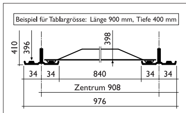
Detailmasse für Tablar MT940
