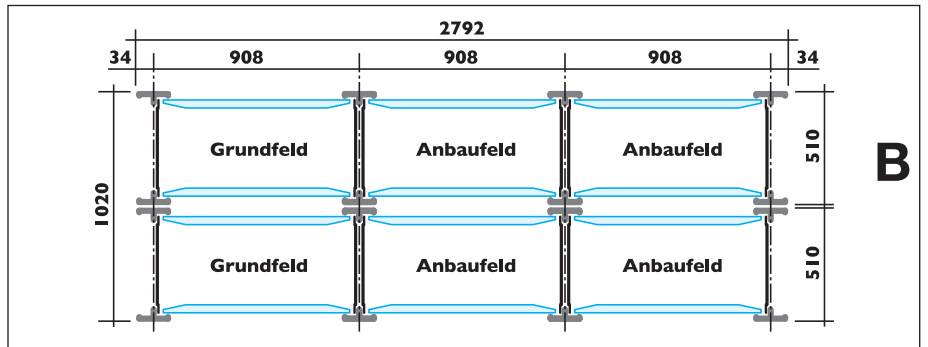
Vermasste Doppelregalreihe zum Definieren der Aussenmasse. Dieses einfache Beispiel zeigt den Hergang einer Planung für Wagen von Verschiebeanlagen! Die Feldlängen sind wichtig für die Produktion der Wagen, damit ein Stützprofil am Wagen für die inneren Rahmen montiert werden kann.
