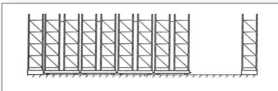
Für Gangbreiten-Angaben der Stapler, siehe Blatt 15.4
