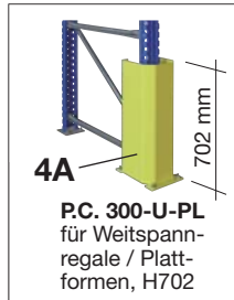
PC. 300 Standard, H300 Anfahrerschutz
